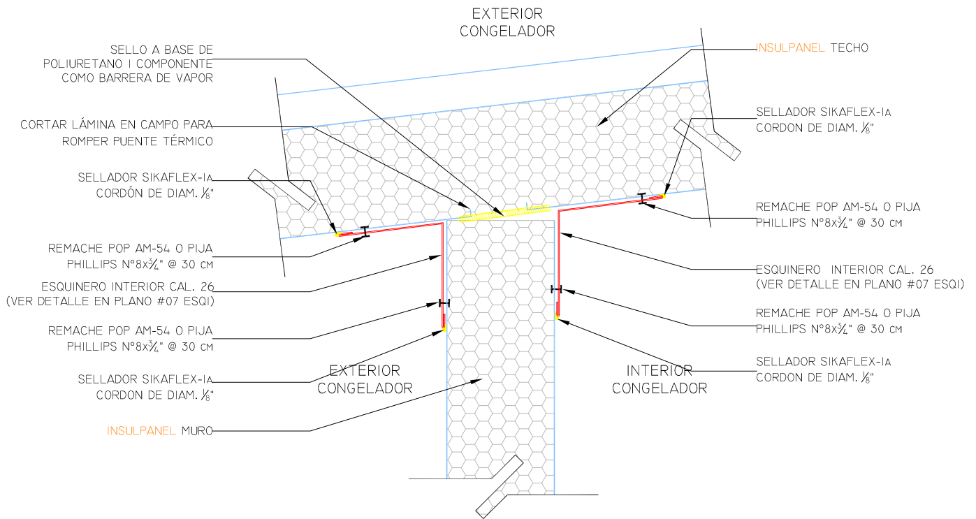
CORTE LONGITUDINAL UNIÓN MURO -CUBIERTA CONGELADOR
