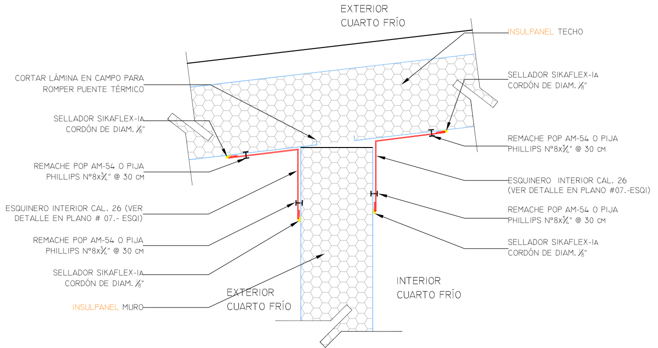
CORTE LONGITUDINAL UNIÓN MURO - CUBIERTA CUARTO FRÍO
